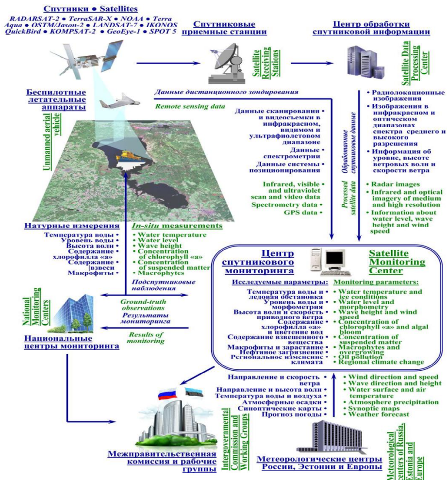
Рис. 1 Обобщенная схема спутникового мониторинга трансграничных водных объектов России и Эстонии [15].
