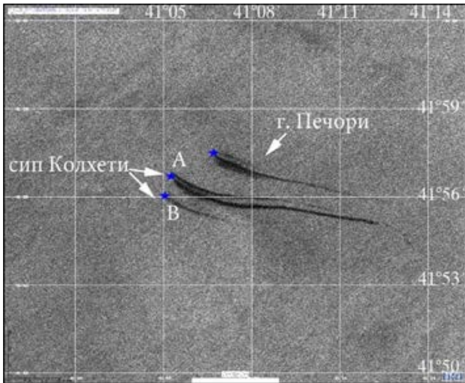
Фрагмент РЛИ SAR Sentinel -1A от 24.05.2016, 03:24 UTC
