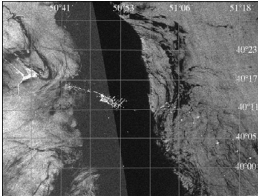
Фрагмент РЛИ ASAR Envisat от 4 июня 2015, 02:43 UTC, полученного над районом нефтедобычи Нефтяные Камни в условиях слабого приповерхностного ветра
