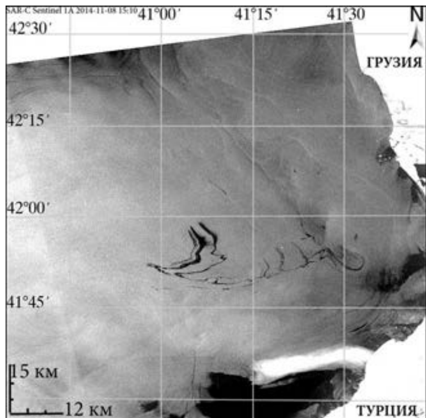
РЛИ SAR Sentinel -1A от 08.11.2014, 15:10 UTC
