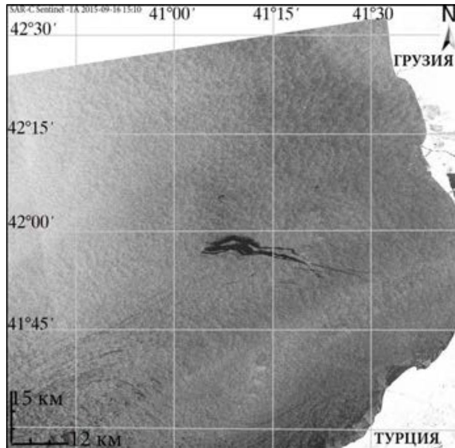
РЛИ SAR Sentinel -1A от 16.09.2015, 15:10 UTC
