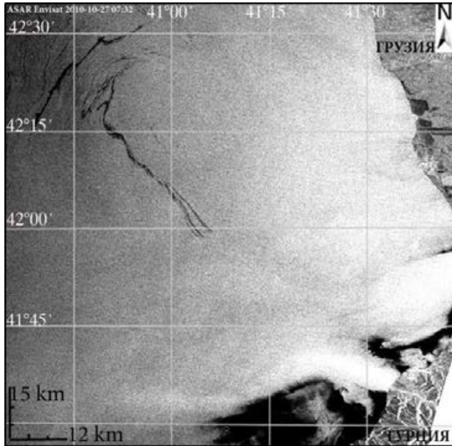
РЛИ ASAR Envisat от 27.10.2010, 07:32 UTC
