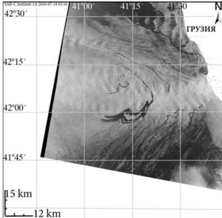
РЛИ SAR Sentinel -1A от 18.07.2016, 03:16 UTC
