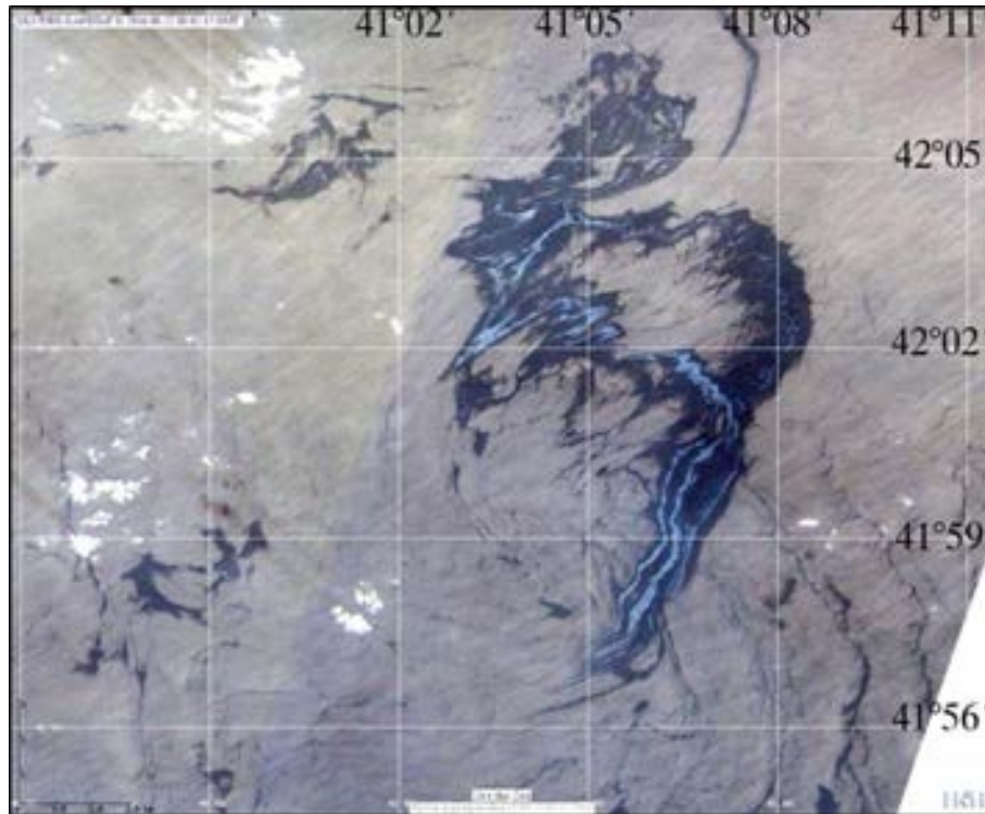
Фрагмент цветосинтезированного изображения сенсора Landsat-8 OLI (4, 3 и 2 спектральные каналы) от 22.08.2016, 08:02 UTC
