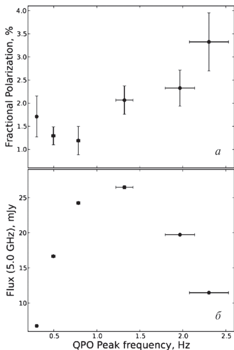
Рис. 8. Зависимость поляризации радиоизлучения (5,0 ГГц) от частоты пика QPO: степень поляризации практически монотонно возрастает с увеличением частоты QPO (а), поток радиоизлучения показывает явную связь с присутствием пика QPO в спектре мощности (б)
