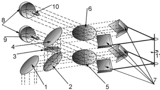
Рис. П1. Оптическая схема блока ПФС-О: 1 — выходное зеркало системы наведения (сканера); 2 — дихроический фильтр; 3 — отрезающий фильтр; 4 — плоское зеркало; 5 — светоделитель ДВК; 6 — светоделитель КВК; 7 — ретрорефлекторы; 8 — параболические зеркала; 9, 10 — детекторы ДВК и КВК соответственно, ЧЭ детекторов находятся в фокальных плоскостях соответствующих параболических зеркал; 11 — ось вращения двухэтажного двойного маятника
