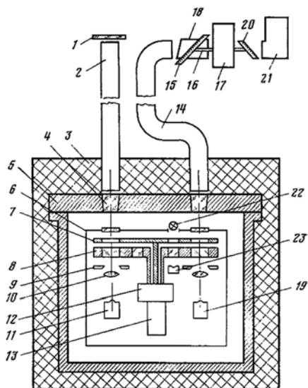
Рис. 4. Схема устройства прибора ИОАВ-2: 1 — молочное стекло; 2 — световод широкоугольного спектрометра; 3 — теплоизоляция; 4 — окно; 5 — герметичная капсула; 6 — опто-электронный узел; 7 — обтюратор модулятора; 8 — КИФ; 9 — щель; 10 — линза; 11 и 19 — фотоприёмники спектрометра; 12 — редуктор двигателя 13; 14 — световод узкоугольного спектрометра; 15 — сканирующее зеркало последнего; 16 — вал двигателя 17; 18 — зеркало; 20 — сканирующее зеркало УФ-фотометра 21; 22 — лампа; 23 — фотоприёмник опорного канала
