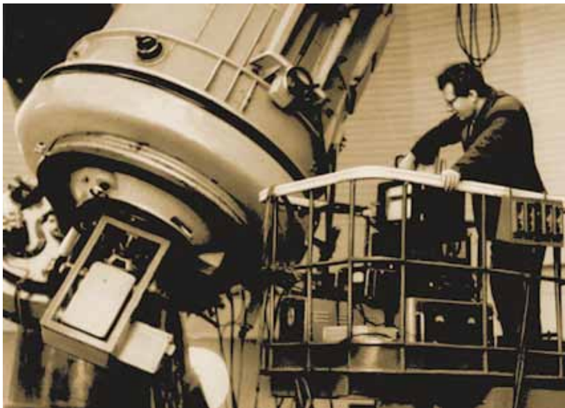
Платформа при телескопе
