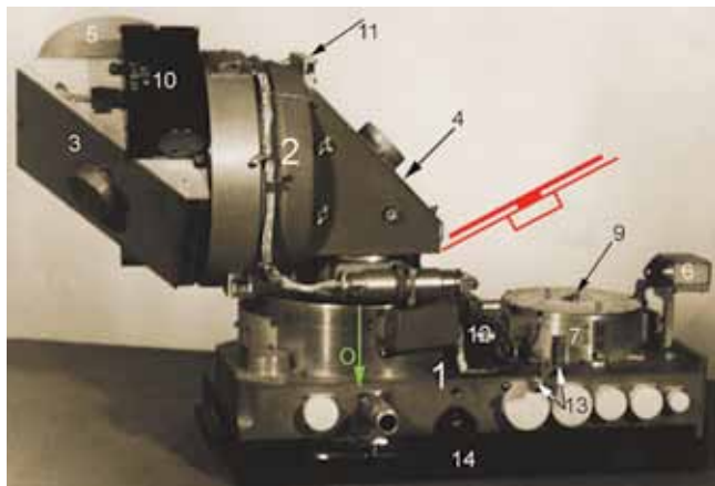
Рис. ПЗ. Сканер (ПФС-С): 1 — неподвижный корпус; 2 — узел вращения зеркал; 3 — входное зеркало; 4 — выходное зеркало; 5 — бленда; 6 — узел арретира вращения сканера; 7 — АЧТ; 8 — многоазовая крышка АЧТ (две её полукруглые створки); 9 — упор разводки створок АЧТ; 10 — торометр; 11 — узел арретира аварийного увода выходного зеркала, условно показано последнее положение последнего после такого «отстрела»; 12 — фиксатор позиционного угла узла выходного зеркала; 13 — одноразовая система съёма и увода крышки торометра; 14 — технологический поддон
