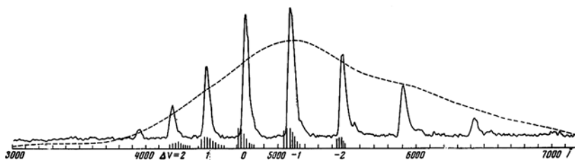
Рис. 2. Зарегистрированное В. А. Краснополяским свечение молекулярного кислорода, состоящее из серии линий O_2
