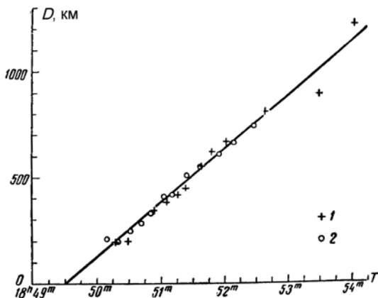
График расширения натриевого облака: 1 — наблюдения В. И. Мороза; 2 — наблюдения В. Ф. Есипова
