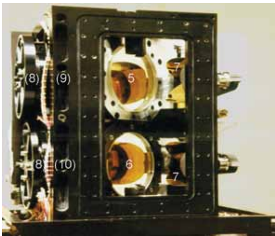
Рис. П2. Вскрытый оптический узел блока ПФС-О. Детекторы и параболические зеркала не видны и их примерные положения показаны условно (в скобках)
