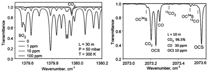
Рис. 3. Примеры спектральных диапазонов и расчётные детали спектра (Н. Игнатьев)
