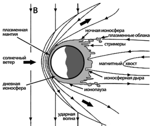
Рис. 6а. Характерные границы и структура взаимодействия Венеры с солнечным ветром
