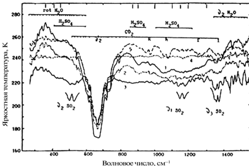
Рис. 6. Примеры спектров теплового излучения Венеры, уходящего в космическое пространство (измерения проводились в 1983 году при помощи фурье-спектрометра на борту «Венеры-15» — одного из советских искусственных спутников планеты); 1 — экваториальная область; 2 — средние широты: 30 < \varphi < 60^\circ \text{ N} ; 3 — холодный «воротник»: 60 < \varphi < 80^\circ \text{ N} ; 4 — полярная область: \varphi > 85^\circ \text{ N} ; 5 — горячий «диполь»: 75 < \varphi < 85^\circ \text{ N} [Zasova et al., 1993]. По таким спектрам определялись на разных широтах вертикальные профили температуры, плотность аэрозольной среды, скорость ветра в средней атмосфере Венеры (~60...90 км), а также содержание \text{H}_2\text{O} и \text{SO}_2 в области верхнего облачного слоя
