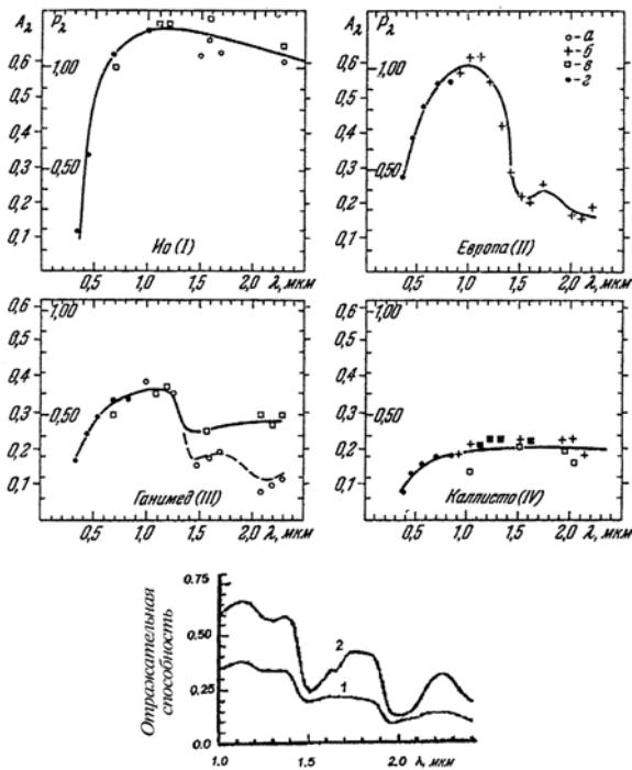
Рис. 1. Вверху: альbedo галилеевых спутников Юпитера в зависимости от длины волны [Мороз, 1965]: наблюдения на ЗТЭ (125-см телескоп Южной станции ГАИШ) в 1963 году (а); наблюдения на ЗТЭ в 1964 году (б); наблюдения на ЗТШ (250-см телескоп Крымской обсерватории АН СССР) (в); UVVRI-фотометрия [Harris, 1961] (г). Спектр отражения Европы показывает сильную полосу поглощения на ~1,5 мкм, характерную для водного льда. Эта полоса, но более слабая, есть и в спектре отражения Ганимеда. Внизу: примеры спектров отражения Европы, полученные через ~30 лет при помощи спектрометра NIMS на космическом аппарате Галилео [McCord et al., 1998]. Спектр 1 относится к области, свободной от ледяного покрова, либо покрытой льдом частично, спектр 2 — целиком покрытой льдом. Среднее между этими двумя спектрами, примерно, соответствует наблюдениям с телескопом. Спектральное разрешение и отношение сигнал/шум в спектрах, полученных при помощи NIMS, было лучше, чем в телескопических. Главным же их преимуществом было, конечно, пространственное разрешение
