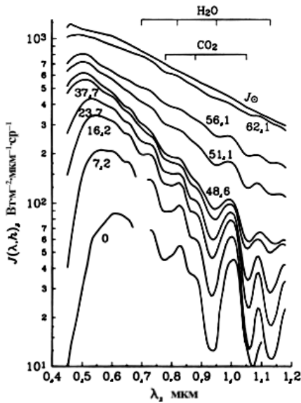
Рис. 3. Примеры спектров многократно рассеянного солнечного излучения в глубоких слоях атмосферы Венеры. Измерения проводились в 1978 году с борта посадочного аппарата «Венера-11» в интервале от 62 км до поверхности. Высота в километрах дана около кривых. Это многократно рассеянное солнечное излучение. Положения сильных полос H_2O и CO_2 отмечены в верхней части рисунка. Измерялась интенсивность излучения, идущего сверху. Она быстро уменьшается при прохождении через облачный слой до пересечения его нижней границы (~49 км). Здесь аппарат входит в более прозрачную часть атмосферы. Ниже 35 км ослабление снова возрастает — по причине газового рэлеевского рассеяния. По таким спектрам были определены полное содержание воды в атмосфере Венеры [Мороз и др., 1979; Moroz et al., 1980] и его вертикальный профиль [Игнатъев и др., 1997].
